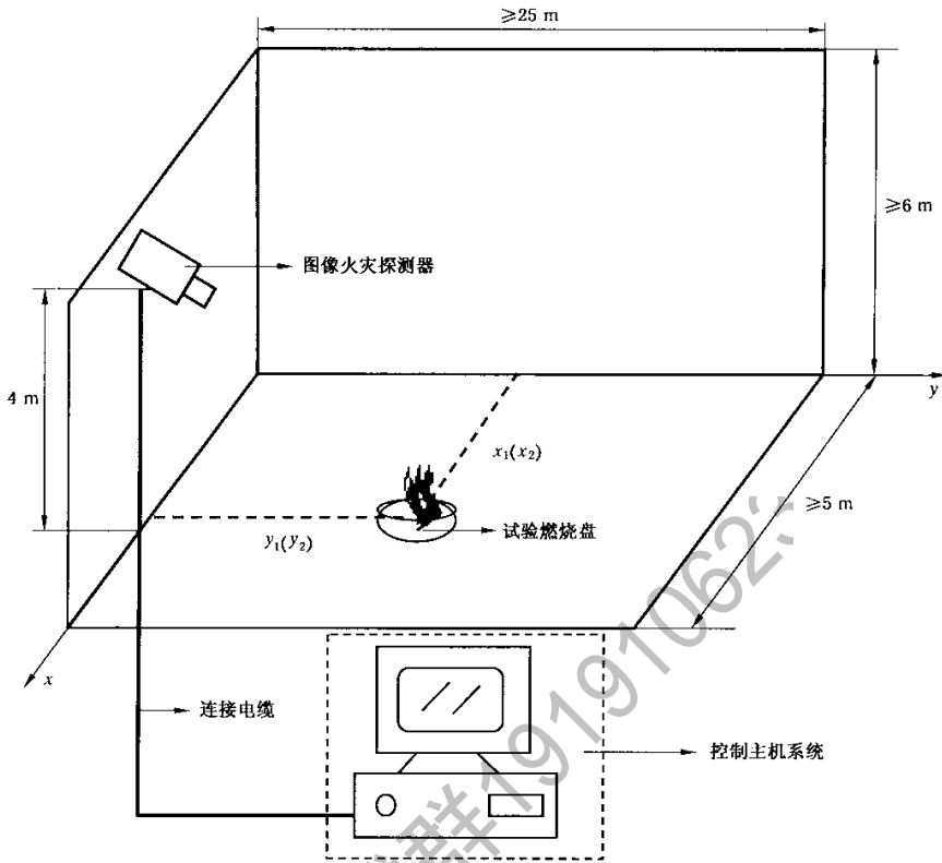
图 4 试验设备和场所示意图
