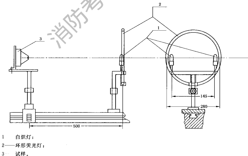
图 5 环境光干扰试验装置结构图
