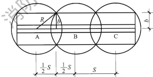
图 7 一股水柱到达任何一点的消火栓布置
